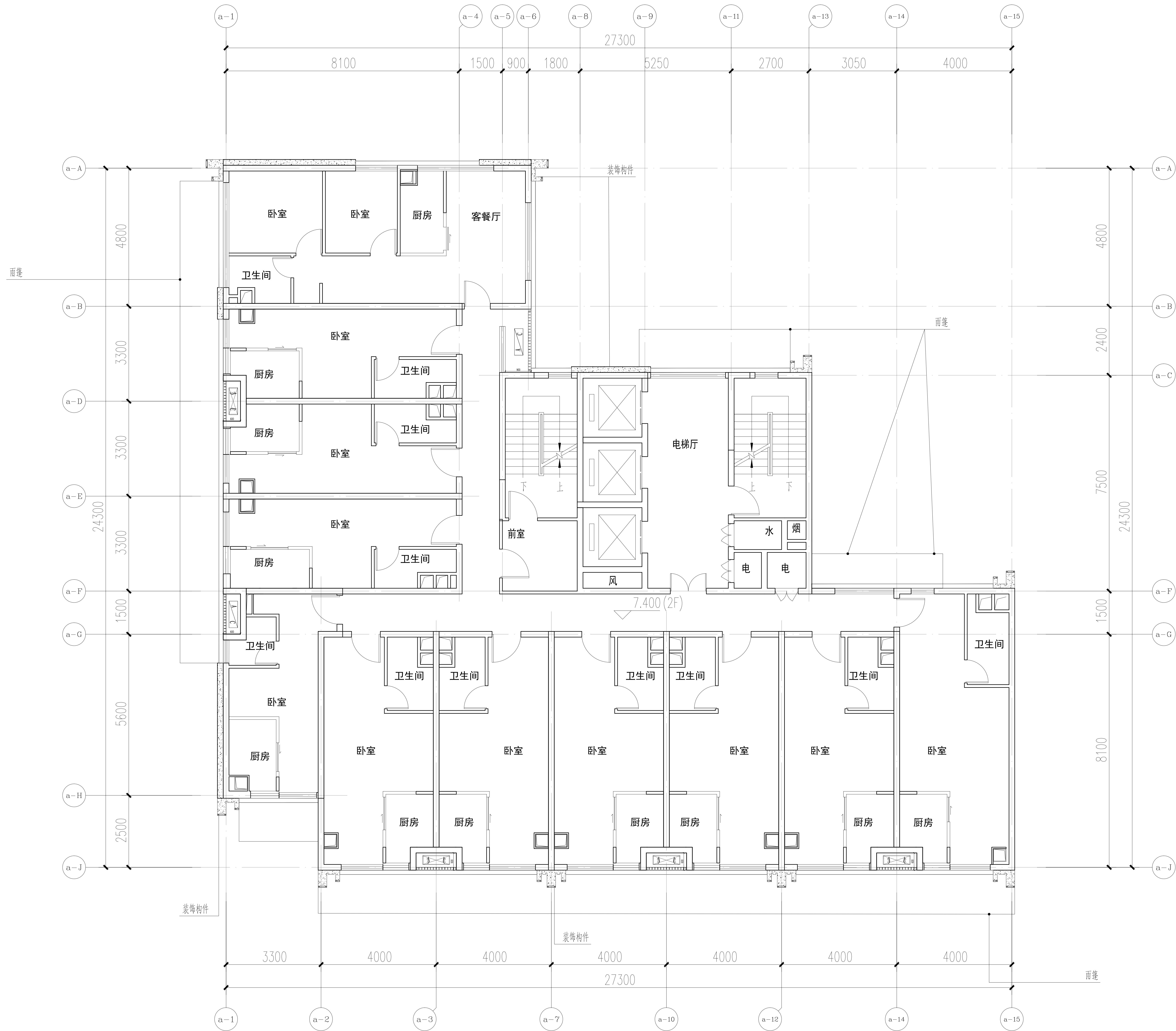
30# 二层平面图 1:100
