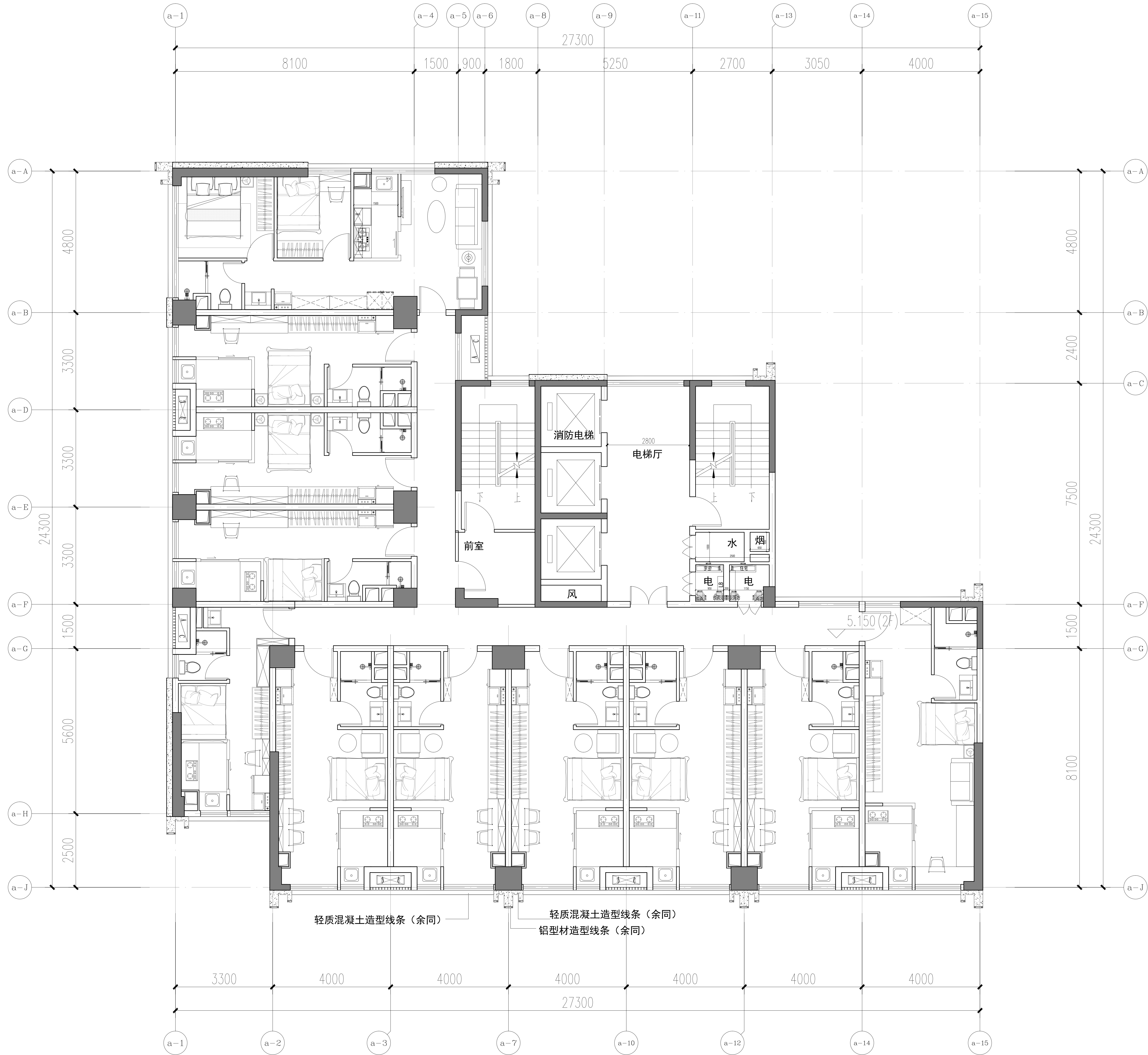
30# 二层平面图 1:100
