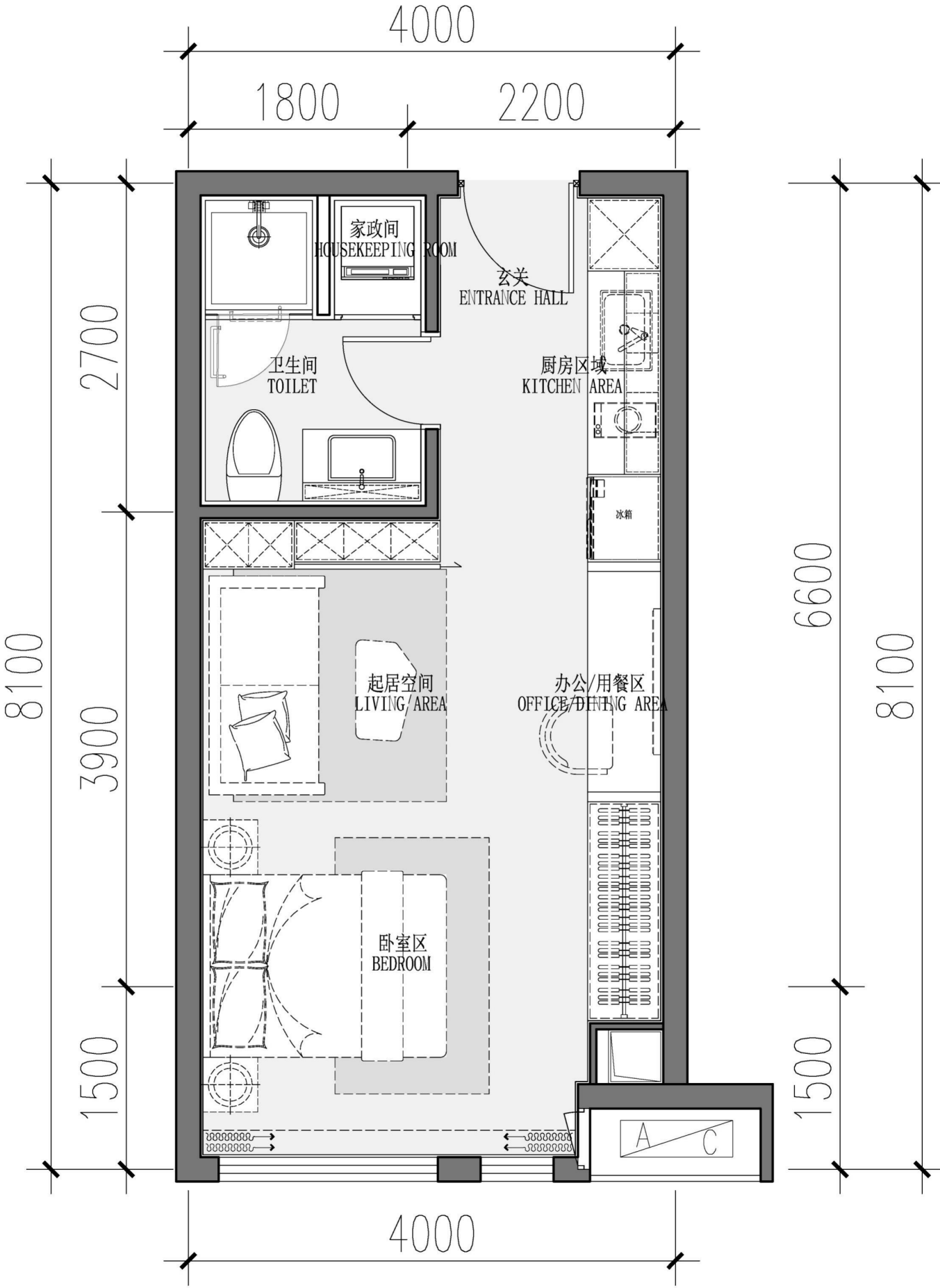
本案45户型平面
